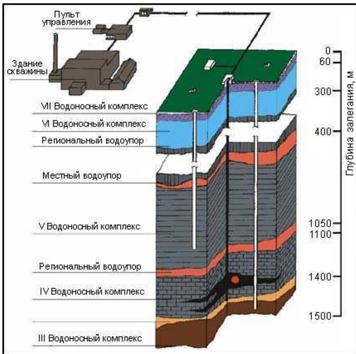
Рисунок 2.8.3-1. Полигон подземного захоронения жидких радиоактивных отходов [138].
