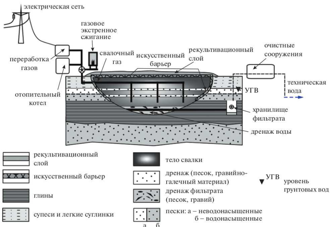
Рисунок 2.8.2-1. Схема строения безопасного полигона в геологическом массиве [135].
