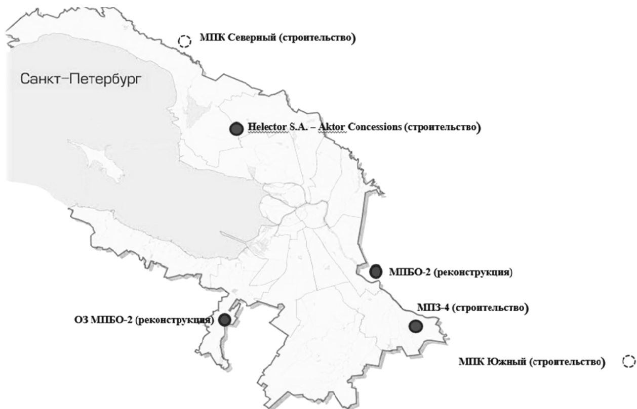
Рисунок 5.2.3-1. Перспективная схема размещения объектов Программы [177].
