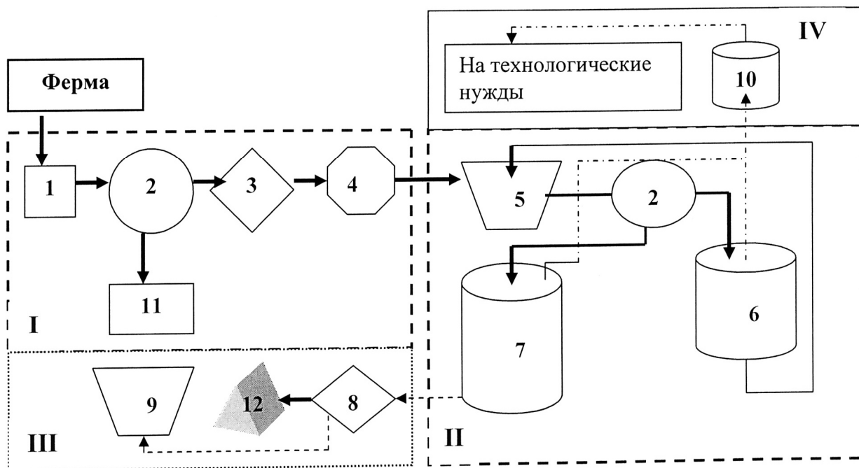
Рисунок 2.6.3-1. Технологическая схема переработки навоза крупного рогатого скота [103]:
