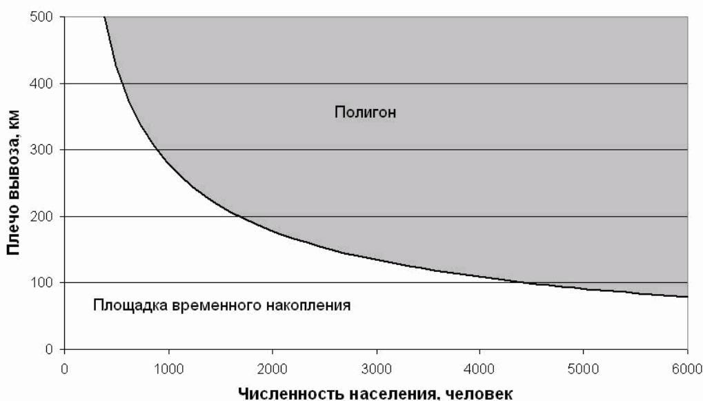
Рисунок 3.1.4-2. Критерий целесообразности строительства полигона или устройства площадки временного накопления [154].
